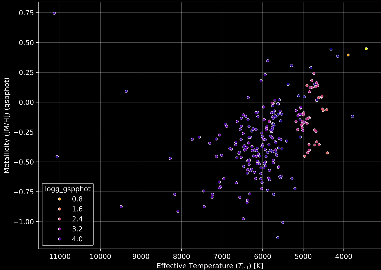
GALAH DR4 Field: [7192] Stellar Population Parameters (n= 237)
